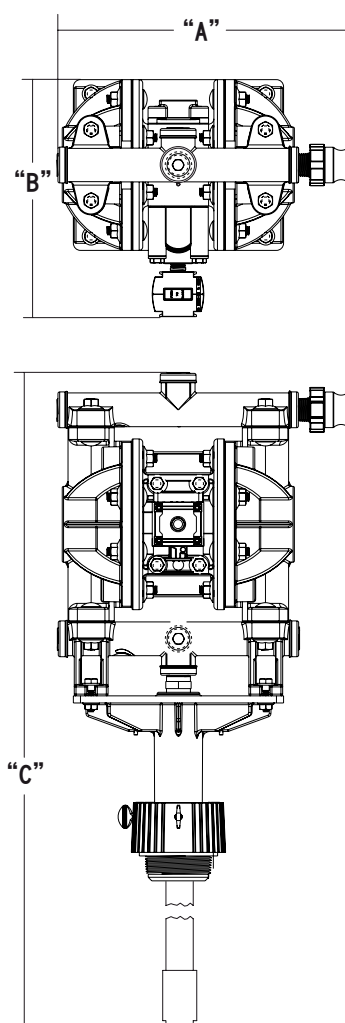
DA005-XXX-X-X 回转泵组件
